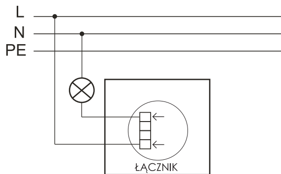
Schemat instalacji łącznika zwiernego.
